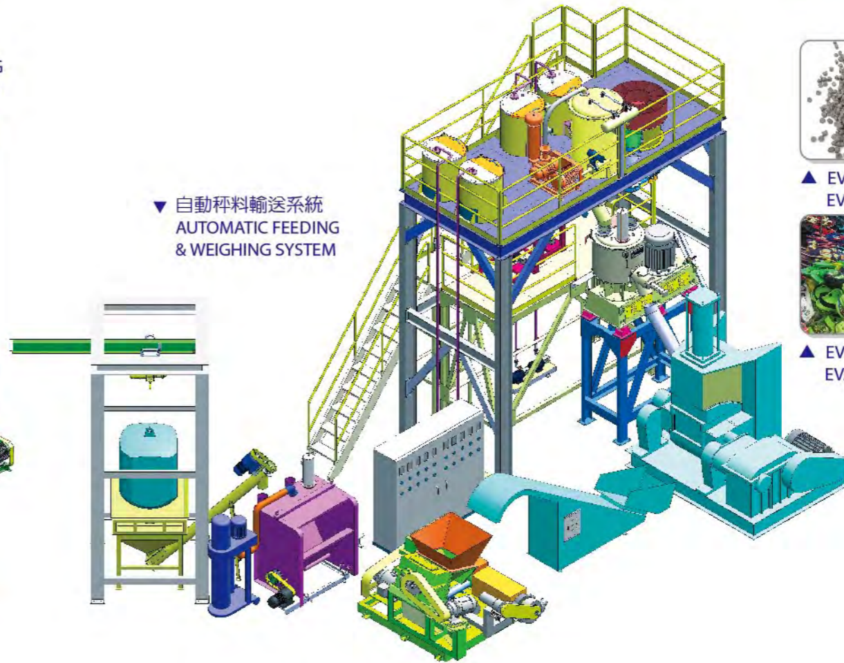
▼ 自動秤料輸送系統 AUTOMATIC FEEDING & WEIGHING SYSTEM
