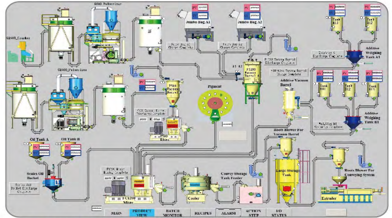
▲ PC電腦控制系統 PC CONTROL SYSTEM
