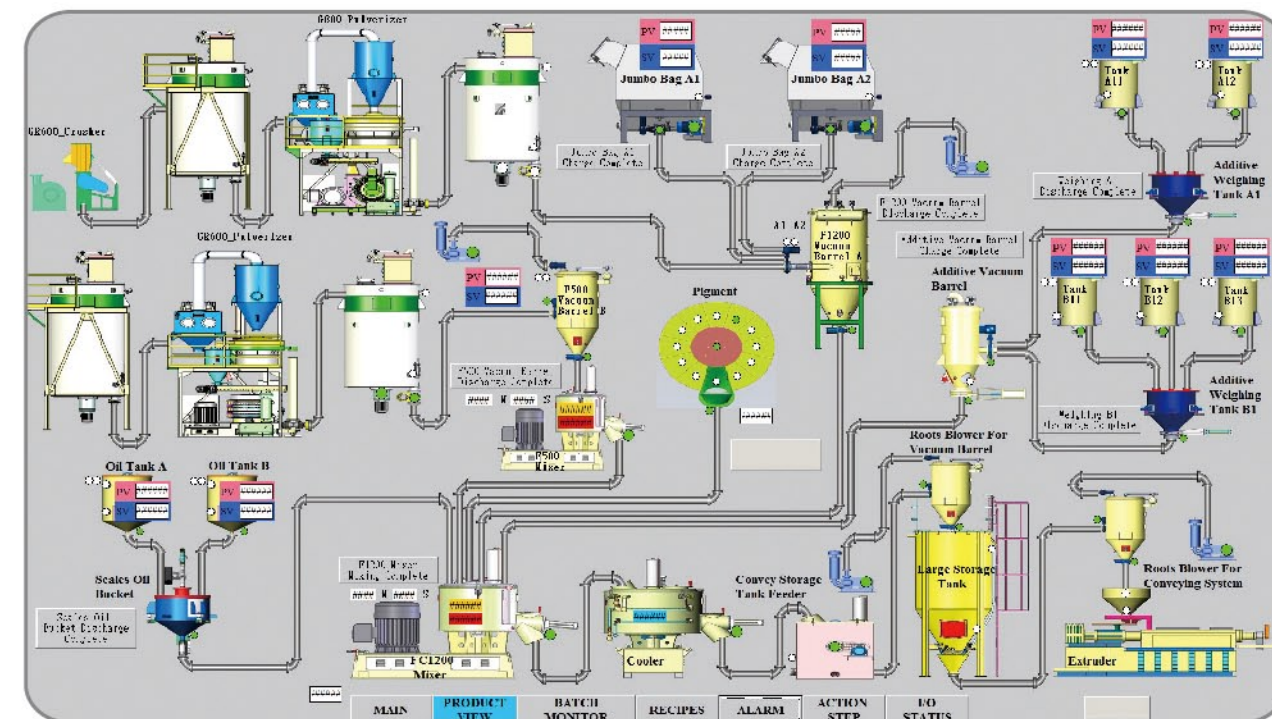
▲ PC電腦控制系統 PC CONTROL SYSTEM
