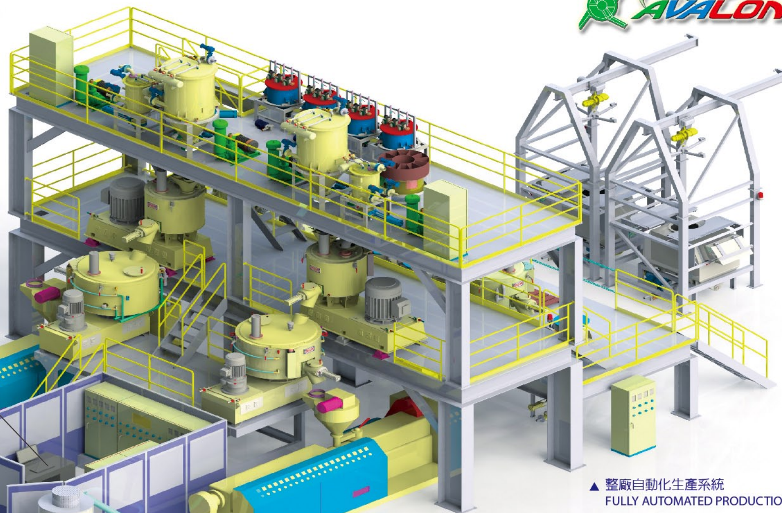
中央電腦控制室 CENTRAL PC CONTROL ROOM
